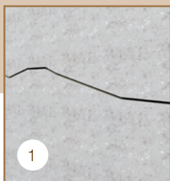
Fisuras en hormigón.
